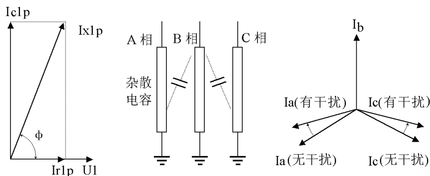
图 8 投影法
